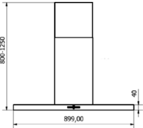
ADAGIO 90 PROFILE40 WANDHAUBE
