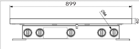
ADAGIO 90 PROFILE40 KOCHFELD
