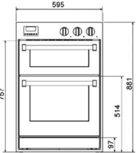
ADAGIO 90 PROFILE40 EINBAUBACKOFEN 60X90
