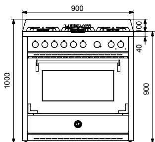
CONCERTO 90
