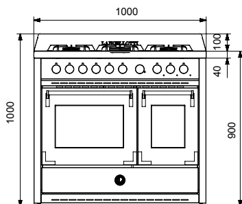
CONCERTO 100
