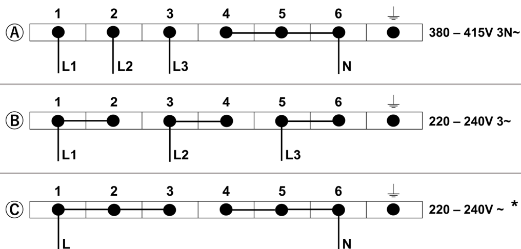
BRANCHEMENT A LA BOÎTE À BORNES
